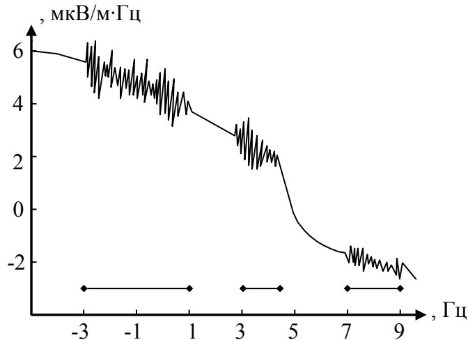
Рис.1.1. Изменение напряжённости электромагнитного поля на поверхности Земли с частотой.
