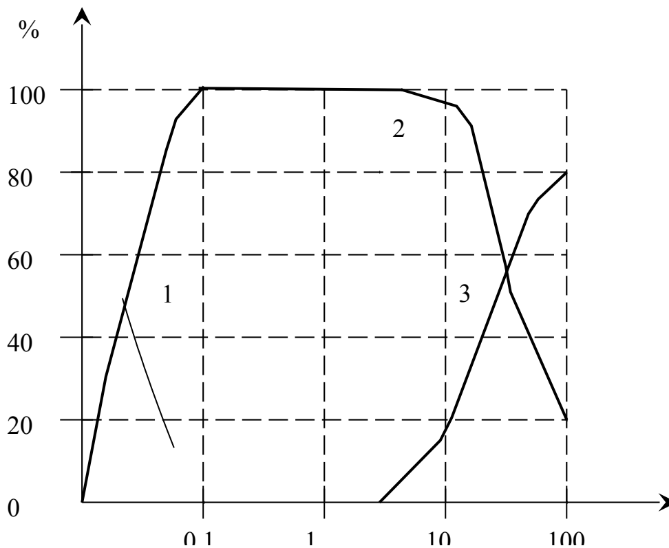
Рис. 3.4 Относительный вклад трех процессов: 1 – фотоэффект; 2 – Комптон – эффект; 3 – образование пар для фотонов различной энергии
