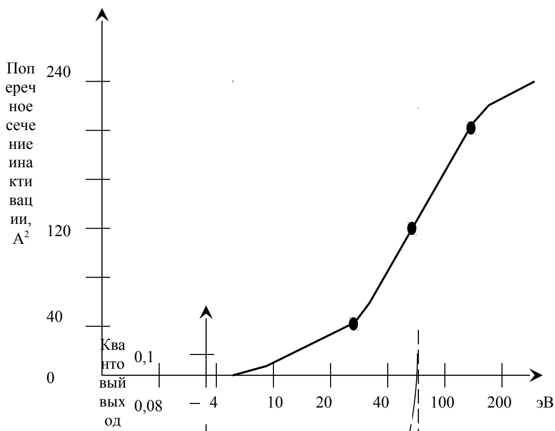
Рис. 3.5 Поперечное сечение инактивации сывальбуина быка от энергии электронов
