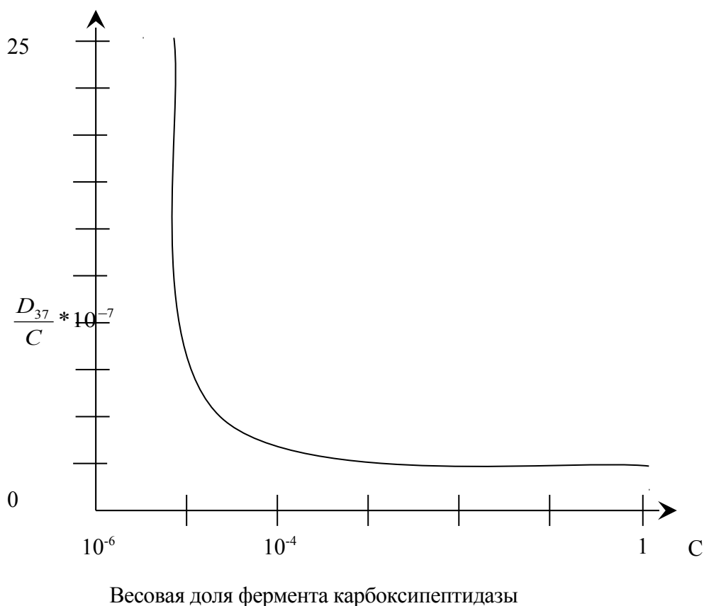
Рис. 3.9. Зависимость инактивирующей дозы D_{37} от концентрации C в области «эффекта разведения» D_{37}/C = \text{const}
