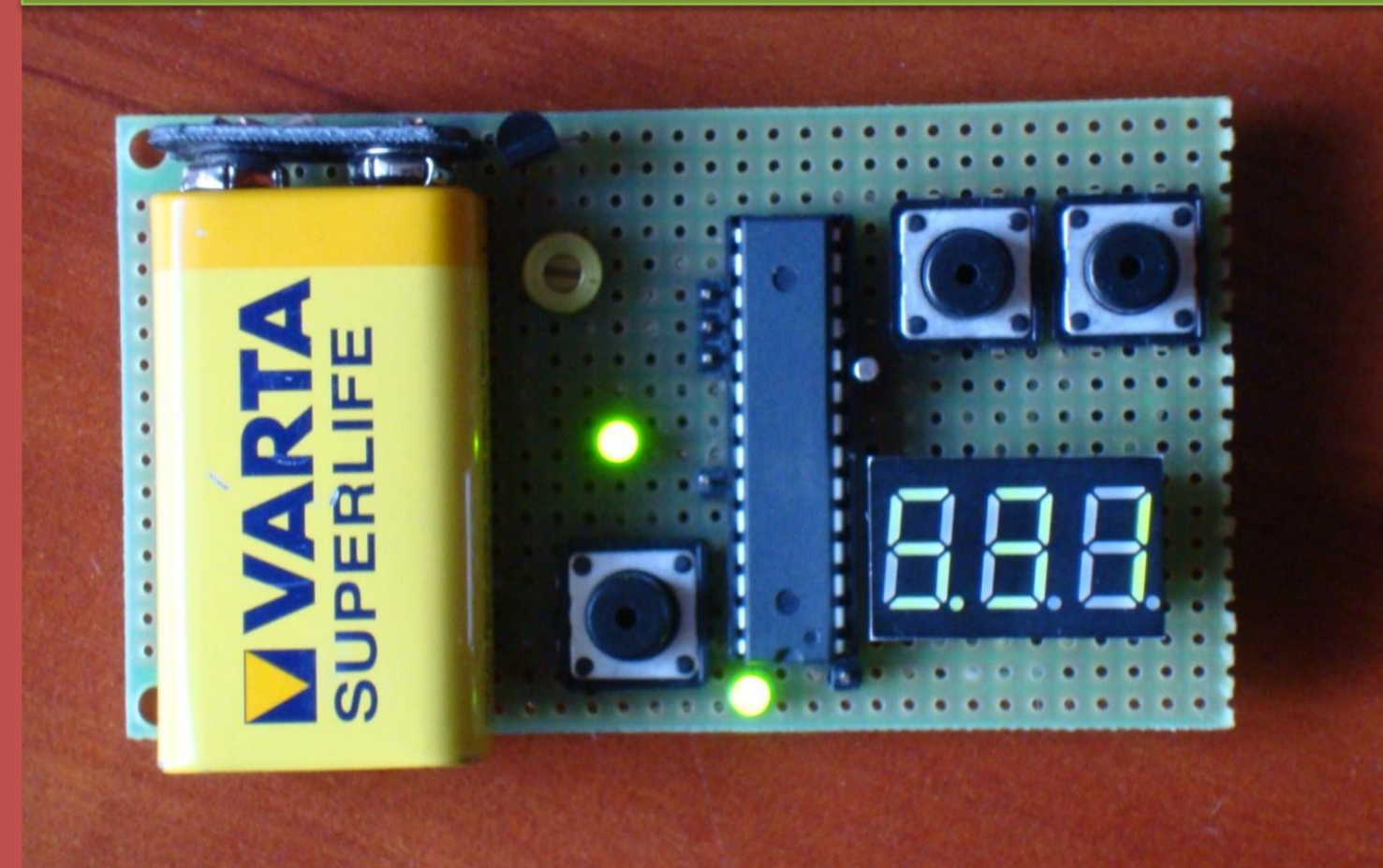
Цифровой таймер обратного отсчета
